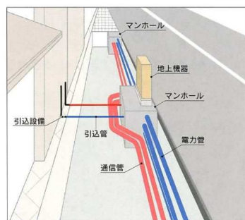
電線共同溝のイメージ
