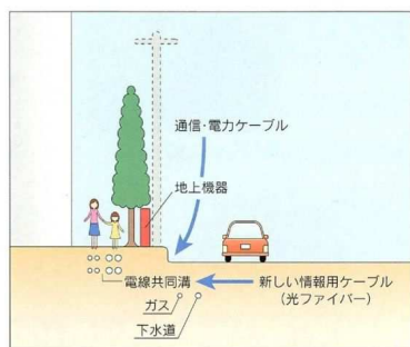
電線共同溝断面イメージ
