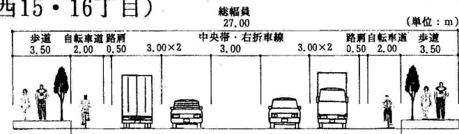
道路の図面 2
